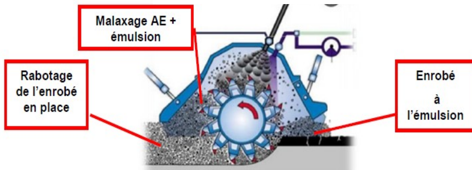
Atelier de retraitement en place ARM 2500 (Source Eiffage Infrastructures) lors d'un chantier sur une route départementale française.
